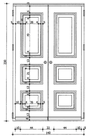
DRZWI WEWNĘTRZNE WAHADŁOWE materiał: drewno dębowe, szkło matowe hartowane
