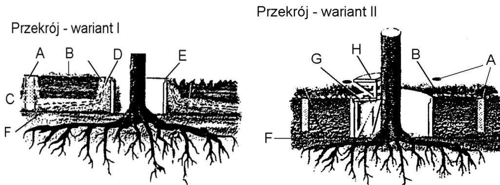
Rys. 5. Studzienka zabezpieczająca pień drzewa przy podwyższeniu terenu powyżej 0,5 m
