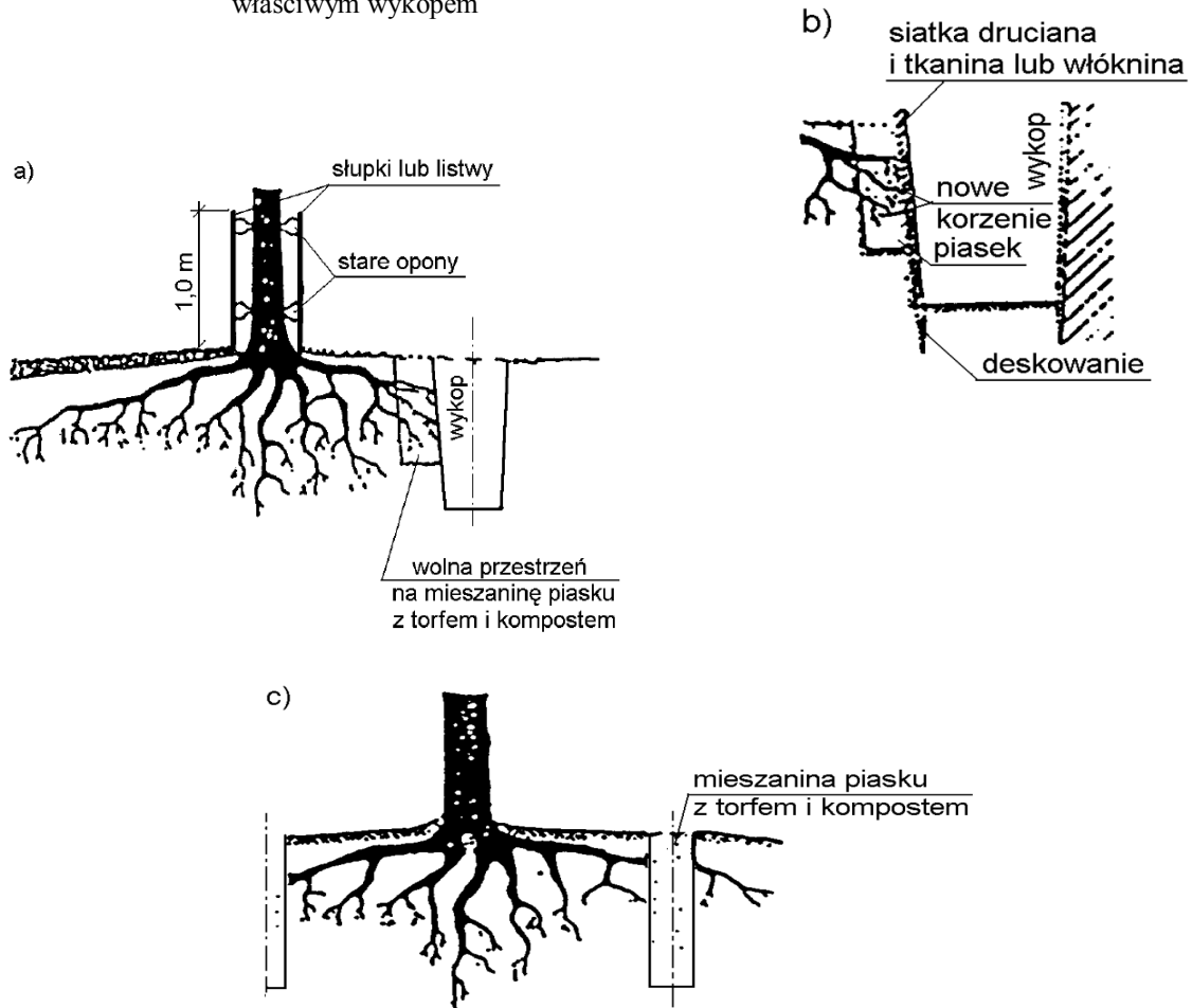
Rys. 2. Zabezpieczenie drzew przy obniżeniu terenu, po wykonaniu wykopów
