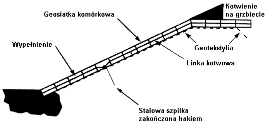
a) Umocnienie skarpy z geosiatką wypełnioną kruszywem
